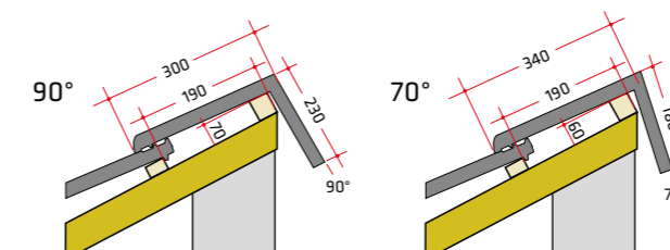
Pultová škridla
