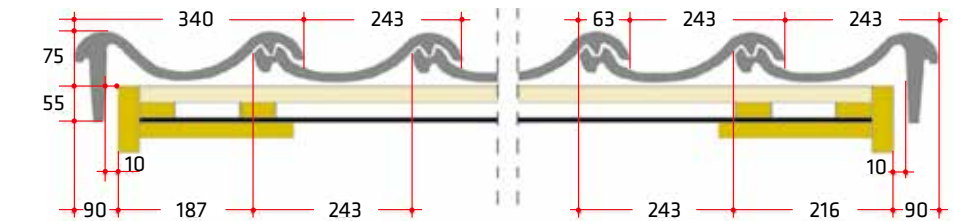
Dachówka skrajna
