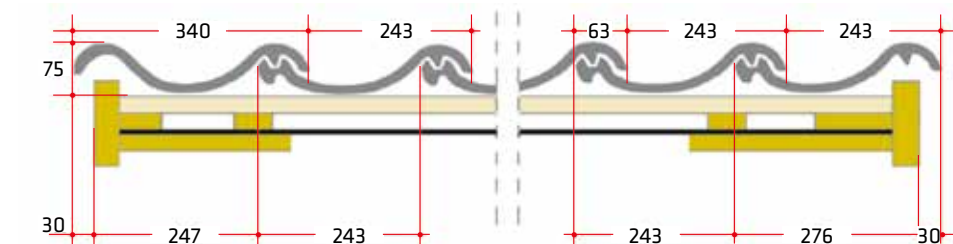
Dachówka dwufalowa
