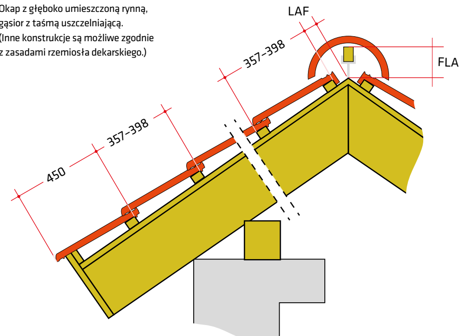
Łaty 30×50 mm
