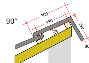
Dachówka pulpitowa
